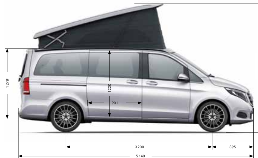
Vue latérale, toit relevable ouvert
