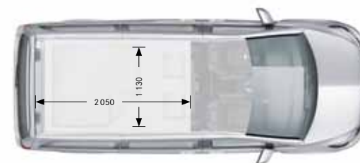
Lit mezzanine dans le toit relevable
